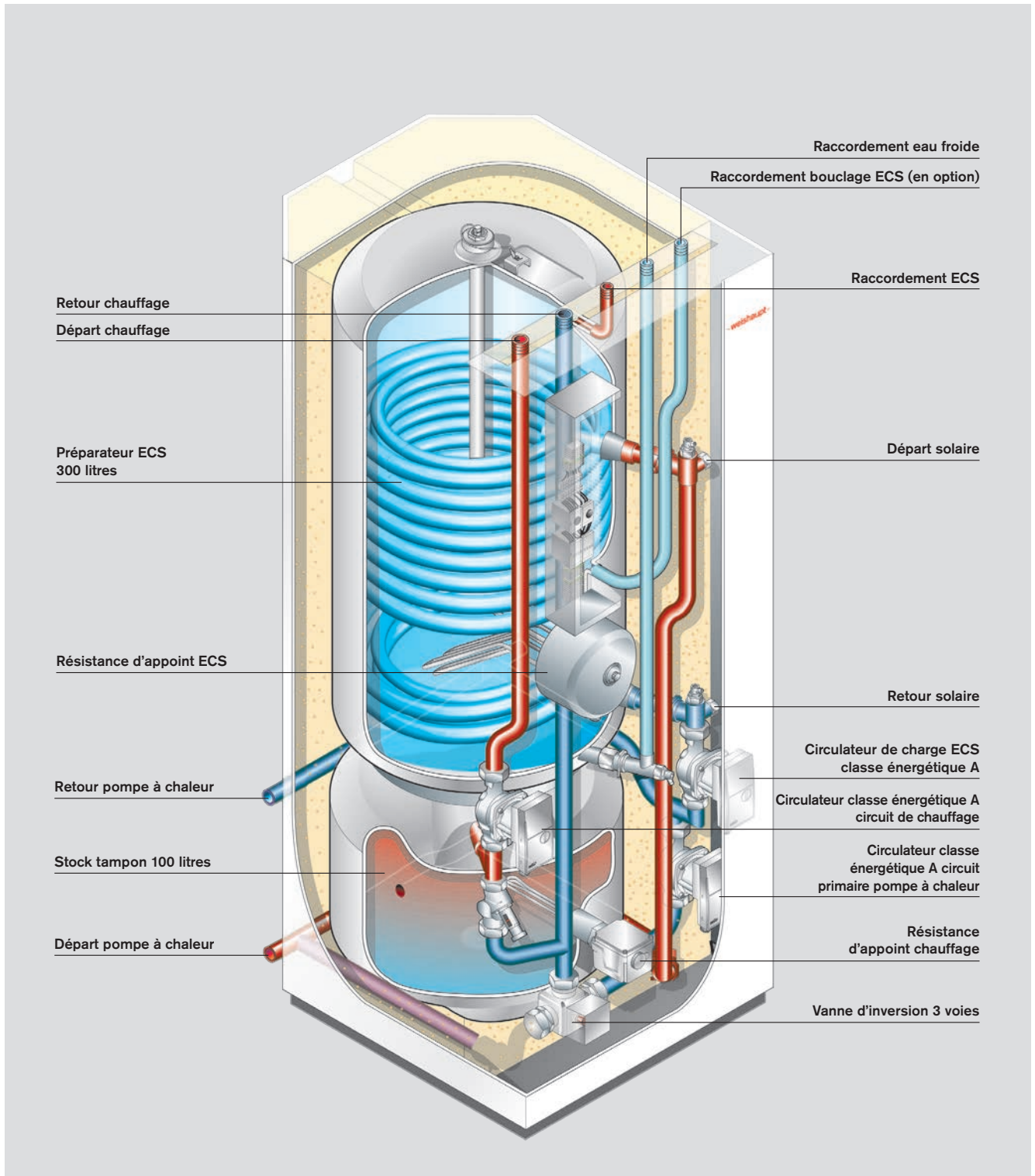
Préparateur multifonction Weishaupt WKS 300 / 100 LE / Unit-E / Bloc / B pour pompes à chaleur monobloc
