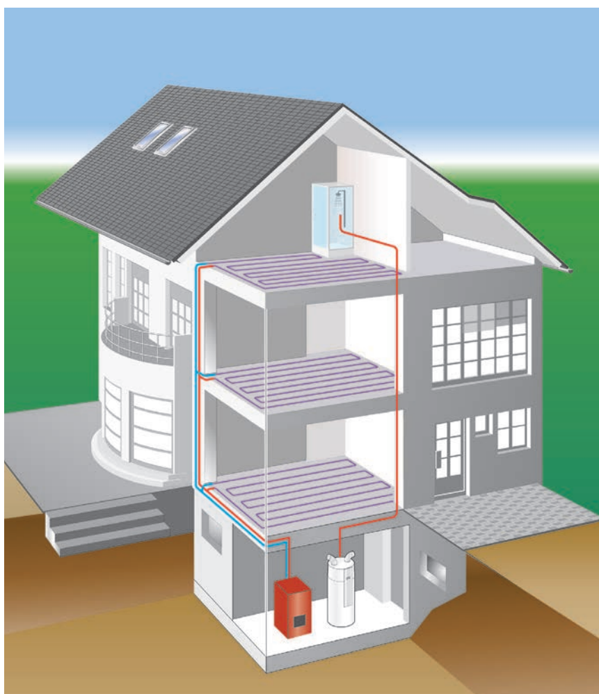
Chauffe-eau thermodynamique
