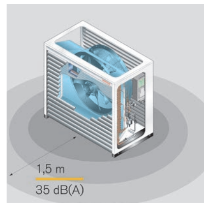
Unité extérieure de la pompe à chaleur bi-bloc WBB 12-A R
